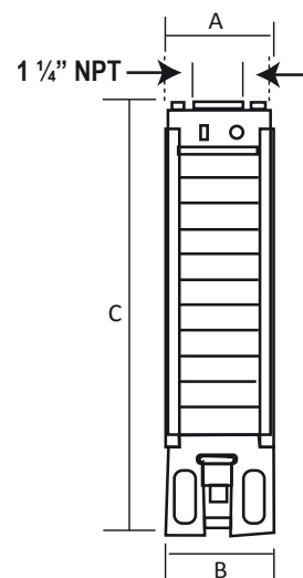
Acoplamiento NEMA 4"
