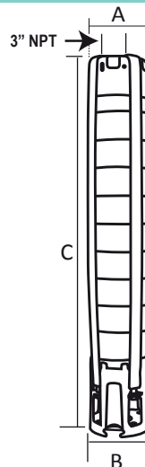
Acoplamiento NEMA 6"
