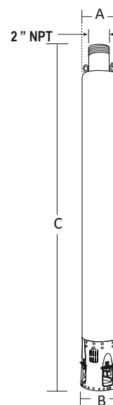
Acoplamiento NEMA 6"
